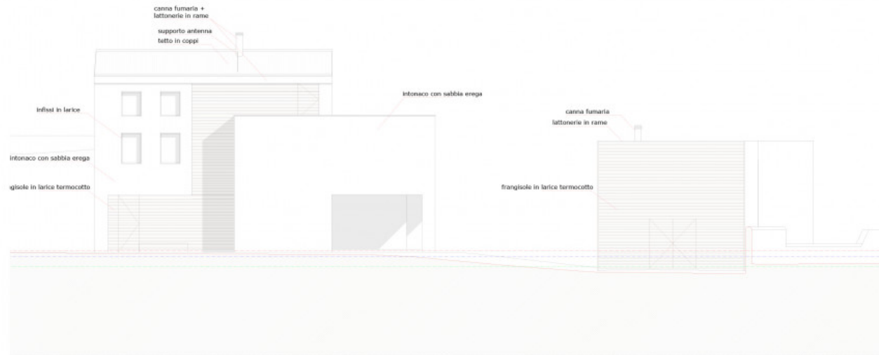
sezione D - D (prospetti)
